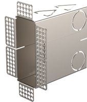
CONTROCASSA DA CAPPOTTO Controcassa zincata LUCIS per cappotto
